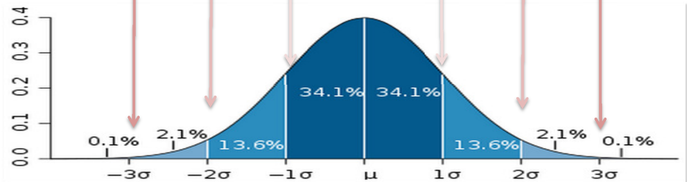
Curva normal / distribuição gaussiana / regra dos 3 sigma
